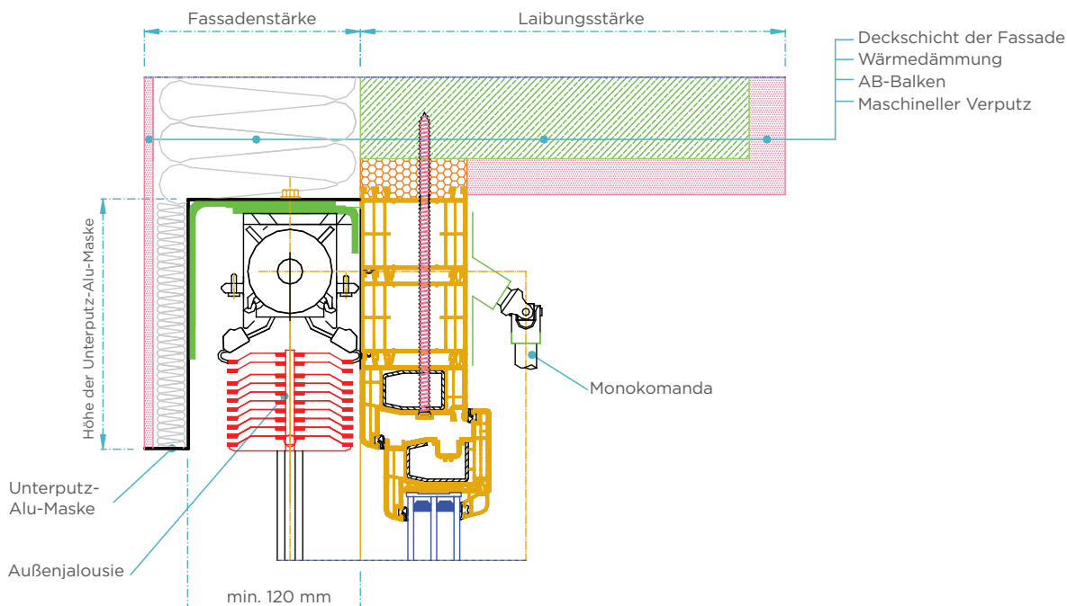
Detail des Fassadenabschlusses am Fensterrahmen mit Außenjalousien. Die Fassade darf nur 5 mm des Kunststoffprofils bedecken.
