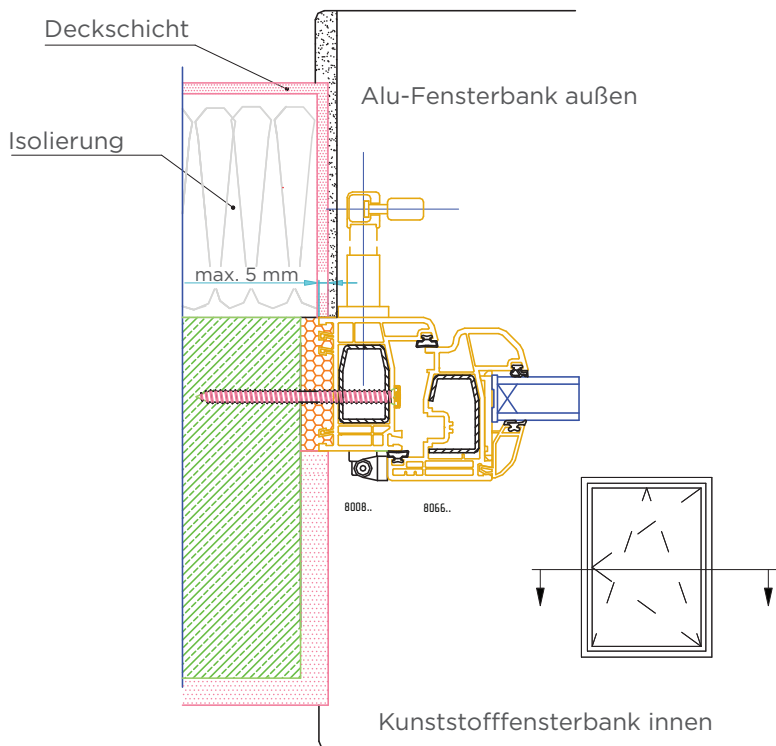
Detail des Fassadenabschlusses am Fensterrahmen mit Außenjalousien. Die Fassade darf nur 5 mm des Kunststoffprofils bedecken.
