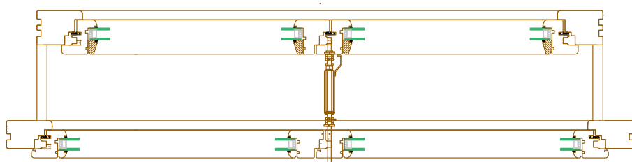
Prez dvokrilnega škatlastega okna s sistemom za odpiranje obeh kril hkrati
