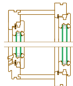
Dvokrilno škatlasto okno s sistemom odpiranja obeh kril hkrati
